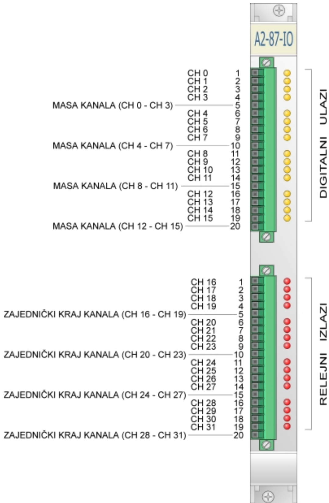
Slika 2.4. Raspored priključaka na priključnim konektorima
