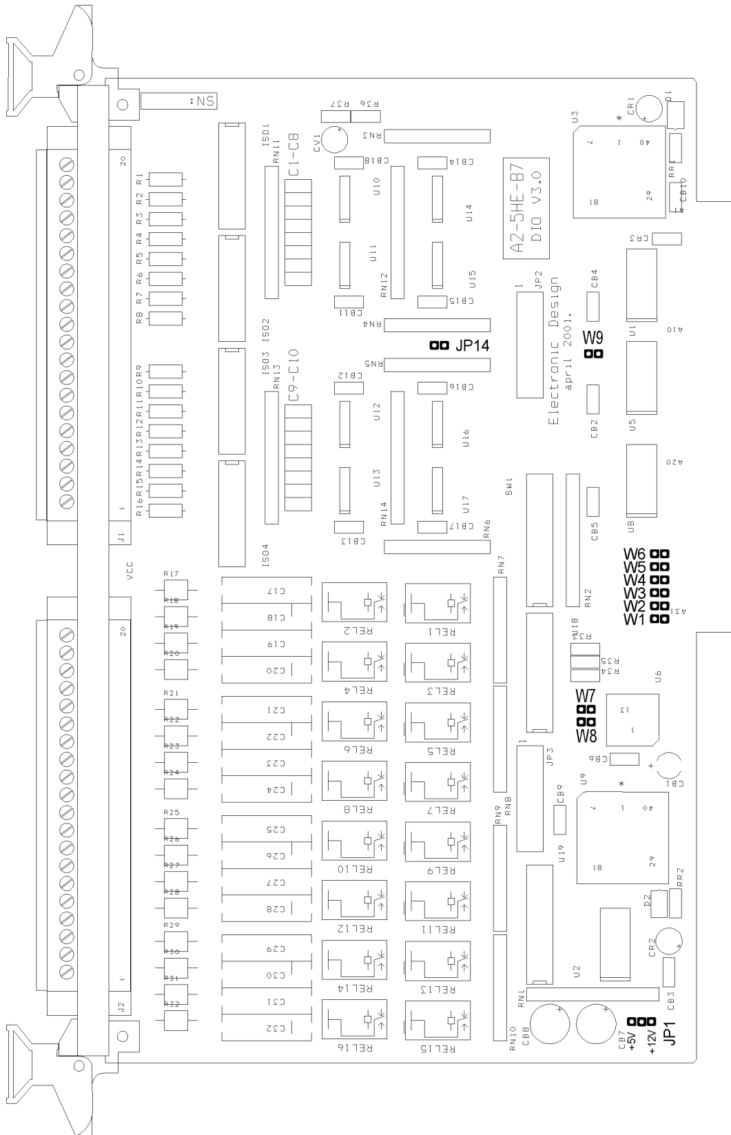
Slika 2.1. Raspored komponenta na modulu A2-87-IO
