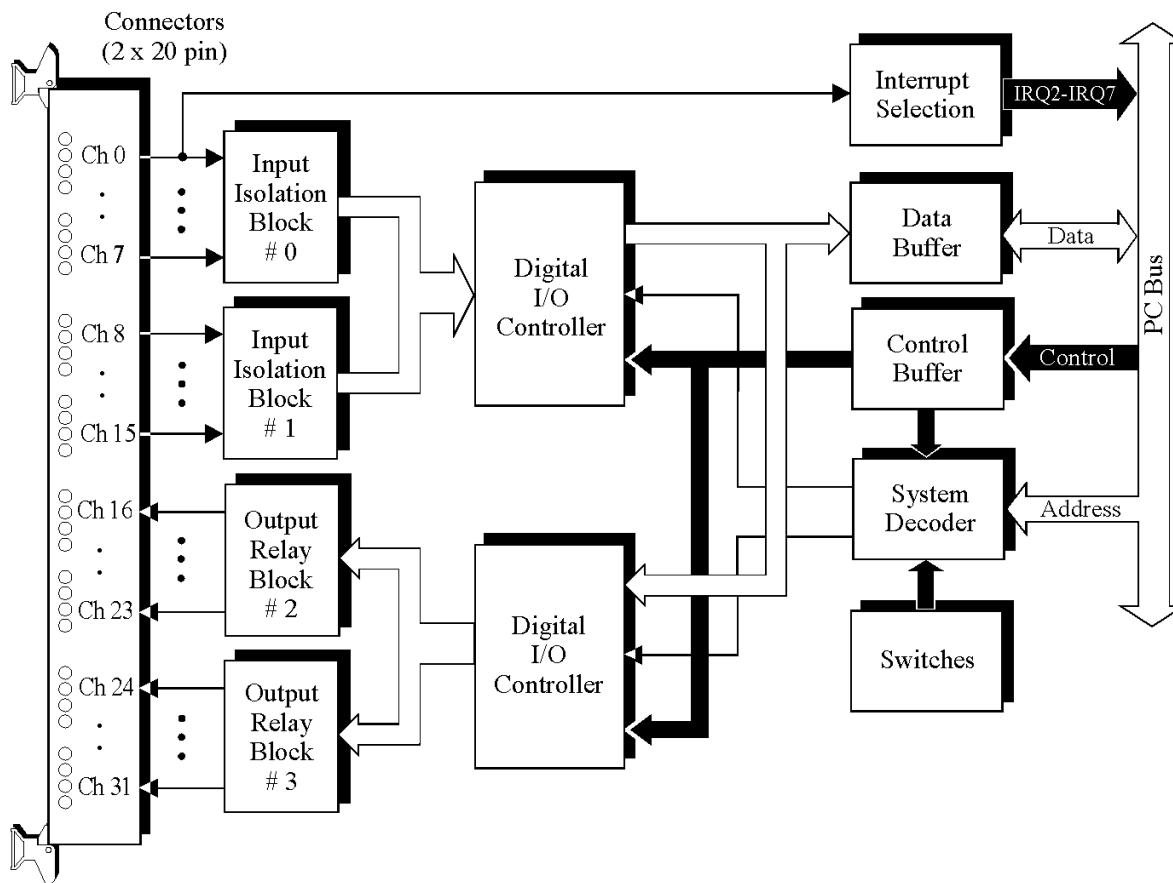
Slika 1.1. Blok-šema modula A2-87-IO
