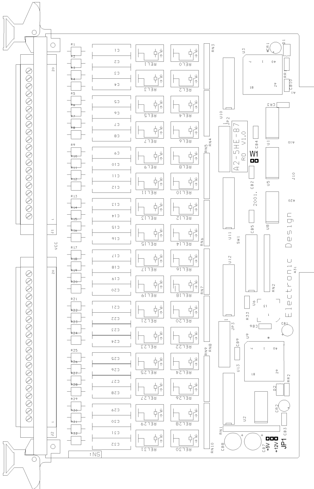
Slika 2.1. Raspored komponenta na modulu A2-87-RO
