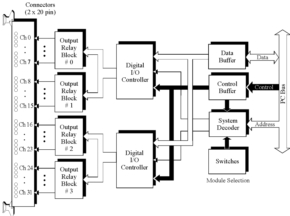
Slika 1.1. Blok-šema modula A2-87-RO
