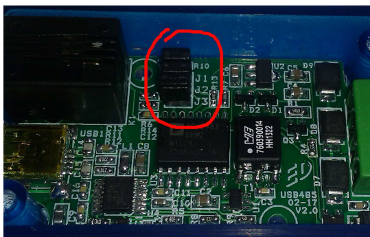
Slika 4. Položaj kratkospojnika
